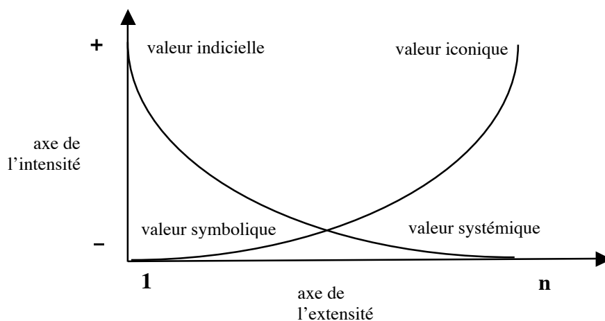
Fig. 1 : Schéma tensif canonique
